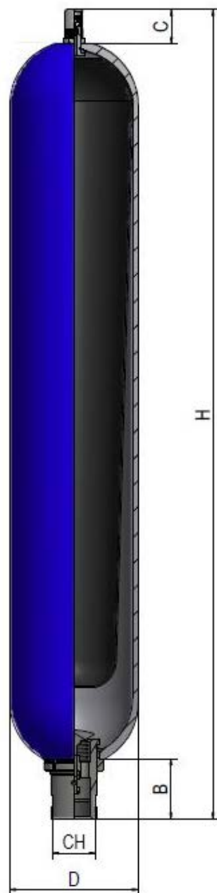
Disegno / Drawing No 1
