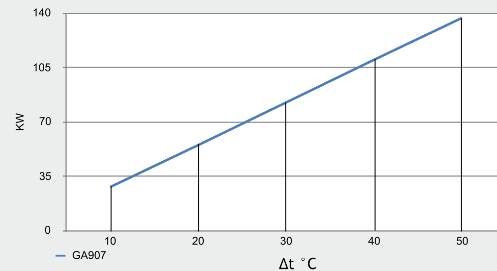
DIAGRAMMA DI RENDIMENTO GA907 - PERFORMANCE DIAGRAM GA907
